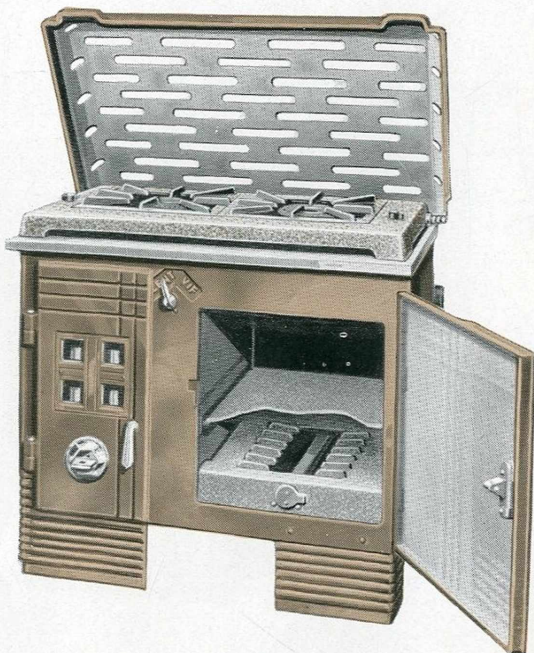
La MIDINETTE B.Z. à gaz. Cheminée cuisinière mixte. Se fait en n°s 1, 2 et 3.
